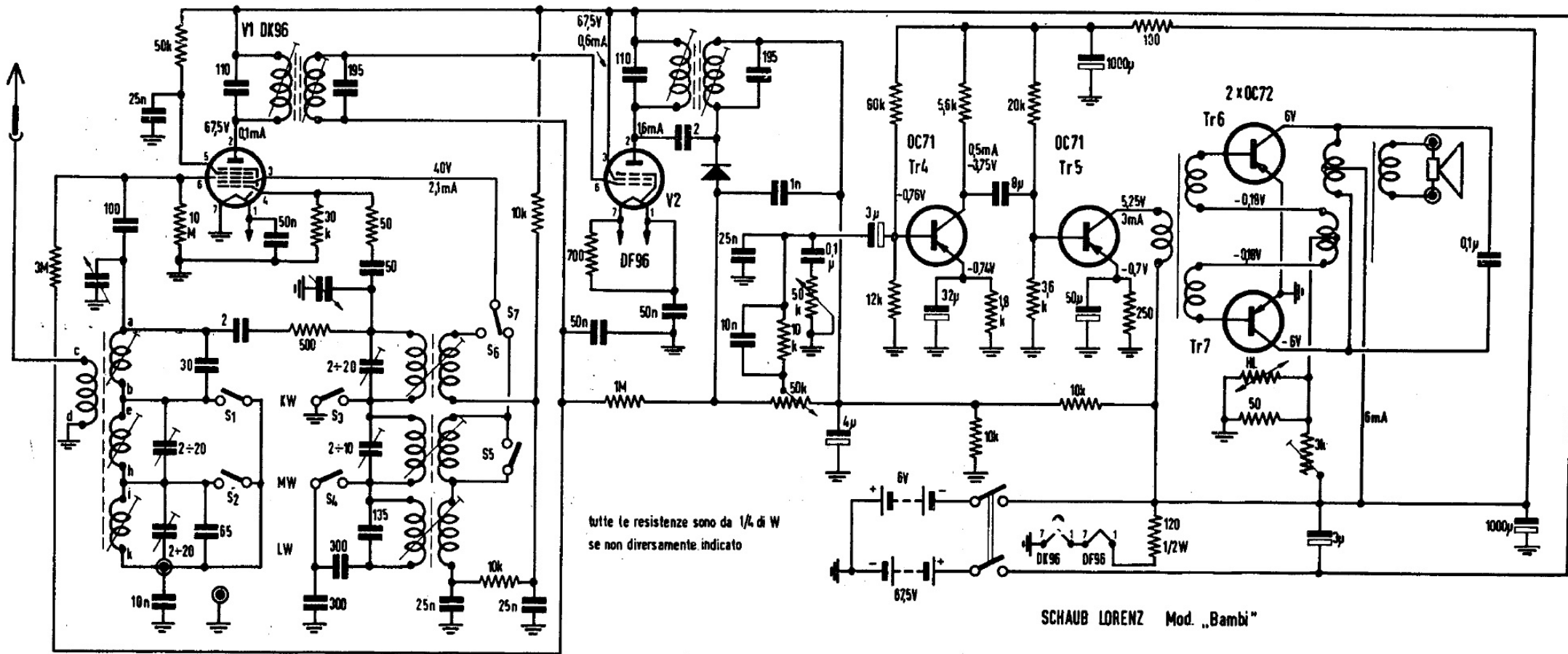
Schema elettrico del radiorecettore SCHAUB LORENZ mod. Bambi
